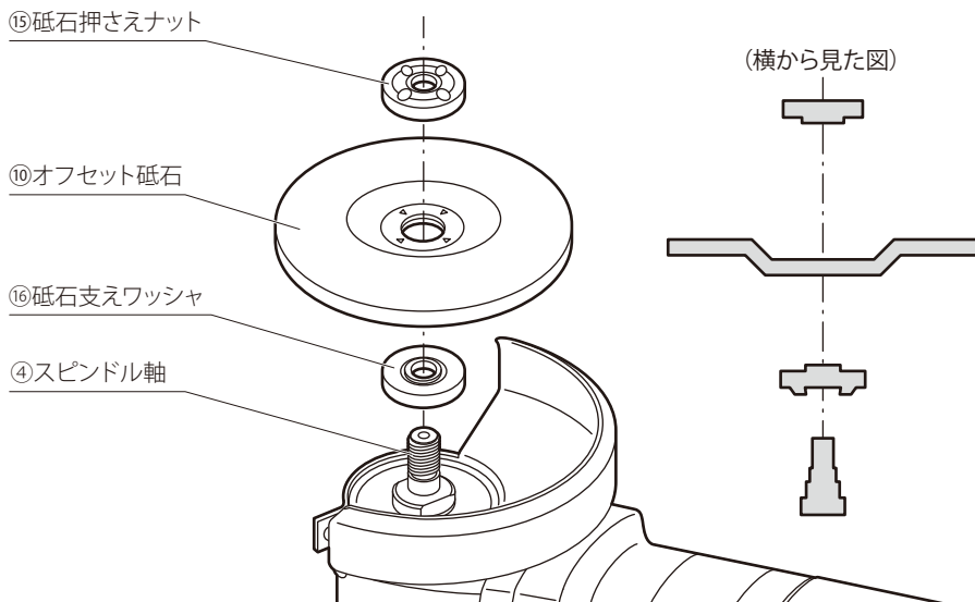
⑮ 砥石押さえナット
